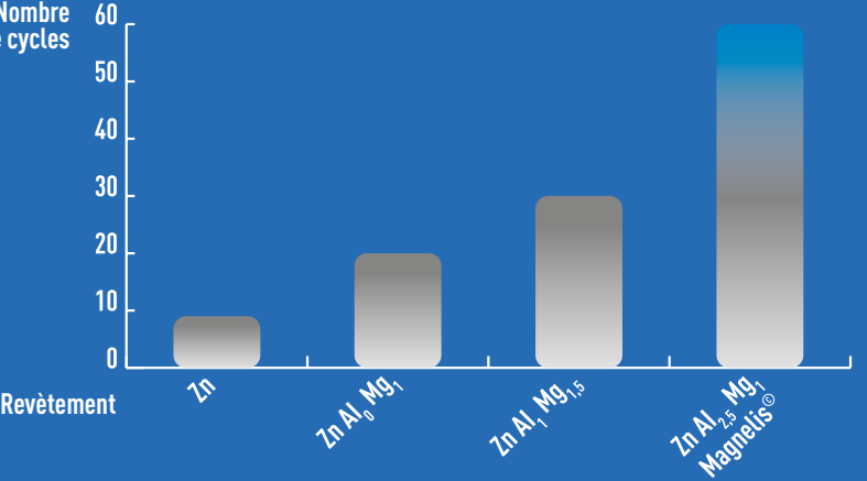
RÉSISTANCE À LA CORROSION DE DIFFÉRENTS REVÊTEMENTS en Zn, Al, Mg au cours d'un test cyclique
